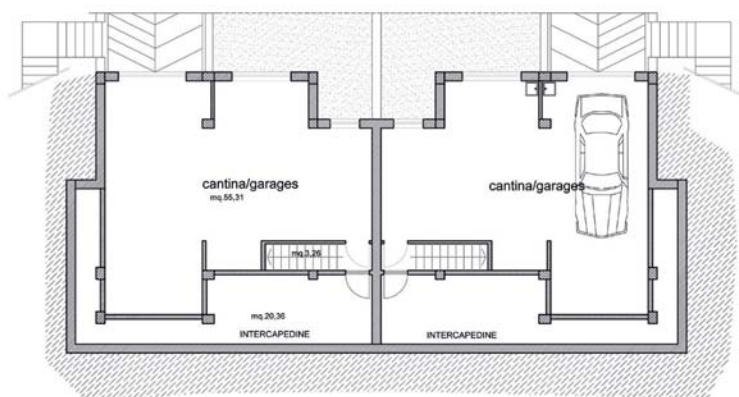
Tipologia "C2" pianta piano interrato
