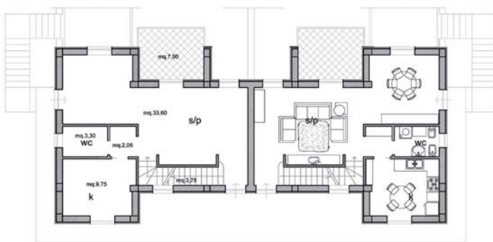
Tipologia "C2" pianta piano terra
