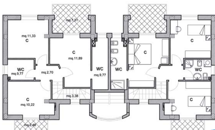
Tipologia "C4" pianta piano secondo
