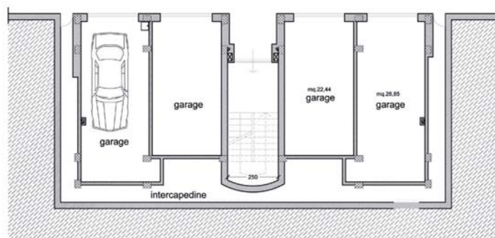
Tipologia "C4" pianta piano interrato tipo
