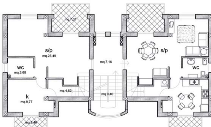
Tipologia "C4" pianta piano primo
